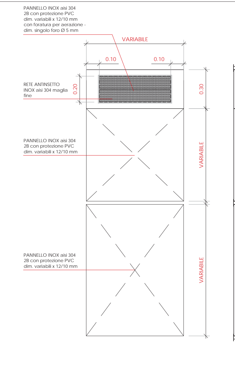
TAMPONAMENTO PORTA: PROSPETTO POSTERIORE E VISTA LATERALE
