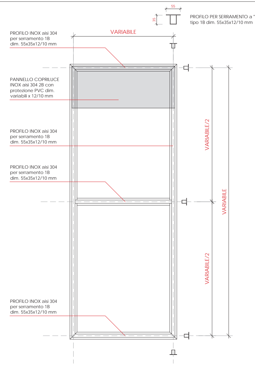
TELAIO PORTA: PROSPETTO POSTERIORE
