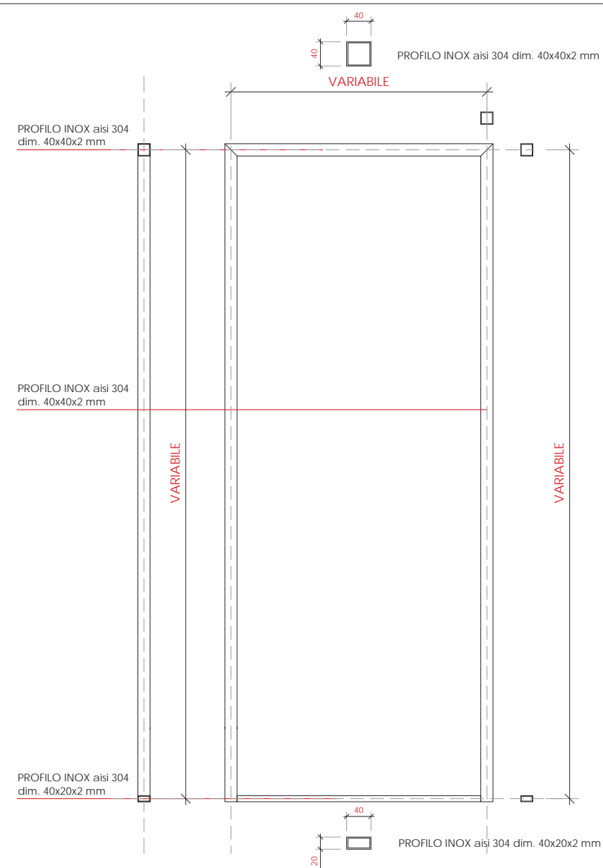
TELAIO ESTERNO: VISTA LATERALE E PROSPETTO
